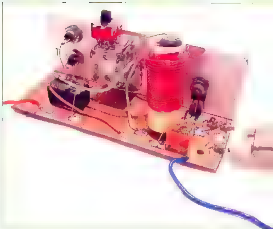
Van links naar rechts: het relais plus de antenne- en ontvanger-aansluitingen, de afstem-C met daarbovenop de schakelaar voor het 160 m-berijk, de spoel, met achter de spoel de aansluiting voor de seinsleutel, de transistor op het aluminium frontje als koeling en tenslotte het kristal in een voetje.
